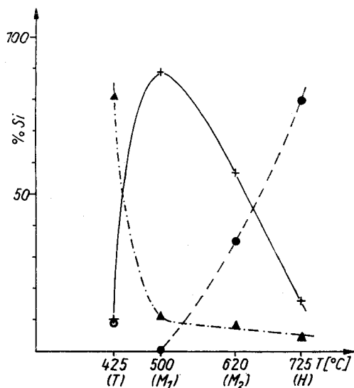
Abb. 2 Silicatanienaufbau der kristallinen Modifikationen des 2\text{PbO} \cdot \text{SiO}_2 (▲ = \Sigma Mono-, Di-, Tri-, + = Cyclotetra-, ● = Poly-, ○ = niedermolekulares Polysilicat)
