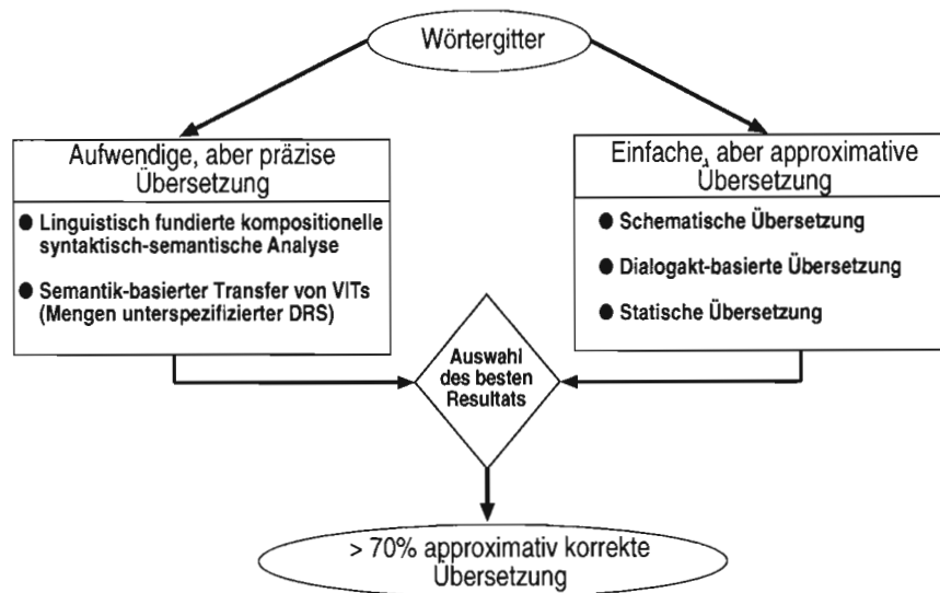
Fig. 2: Die Kombination flacher und tiefer Übersetzungsverfahren
