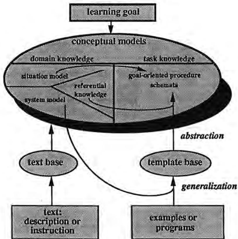
Abbildung 8: Allgemeine Inferenzstruktur des KIWi-Modells (nach Schmalhofer et al., 1993).
