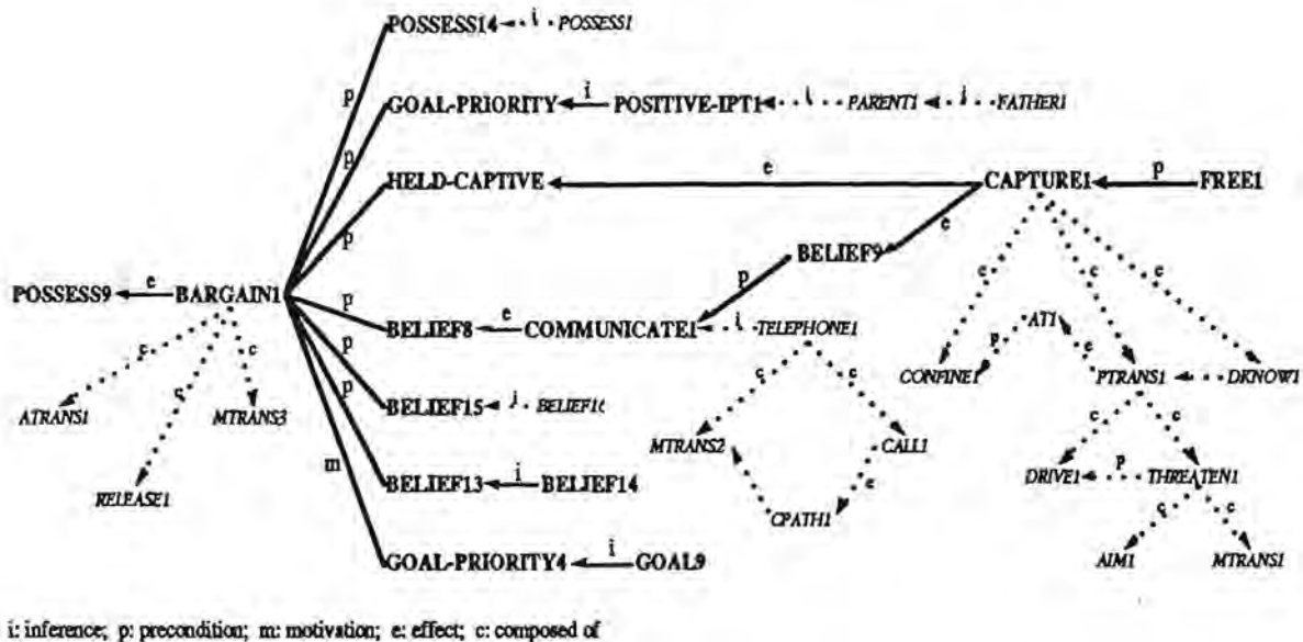
Abbildung 3: Gezeigt ist die vollständige Erklärungsstruktur der Entführungsgeschichte (alle Kanten und Knoten), als auch die generalisierte Erklärungsstruktur (nur fettgedruckte Kanten und Knoten). Die Beschreibungen der einzelnen Knoten sind in Tabelle 1 angegeben (nach DeJong & Mooney, 1986).
