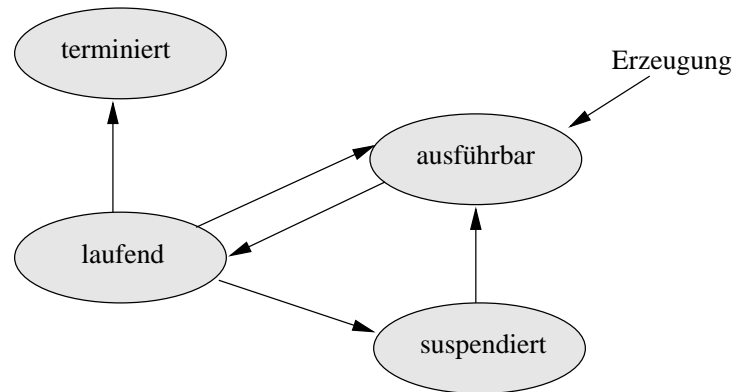
Abbildung 2.6 Zustände und Zustandsübergänge von Threads
